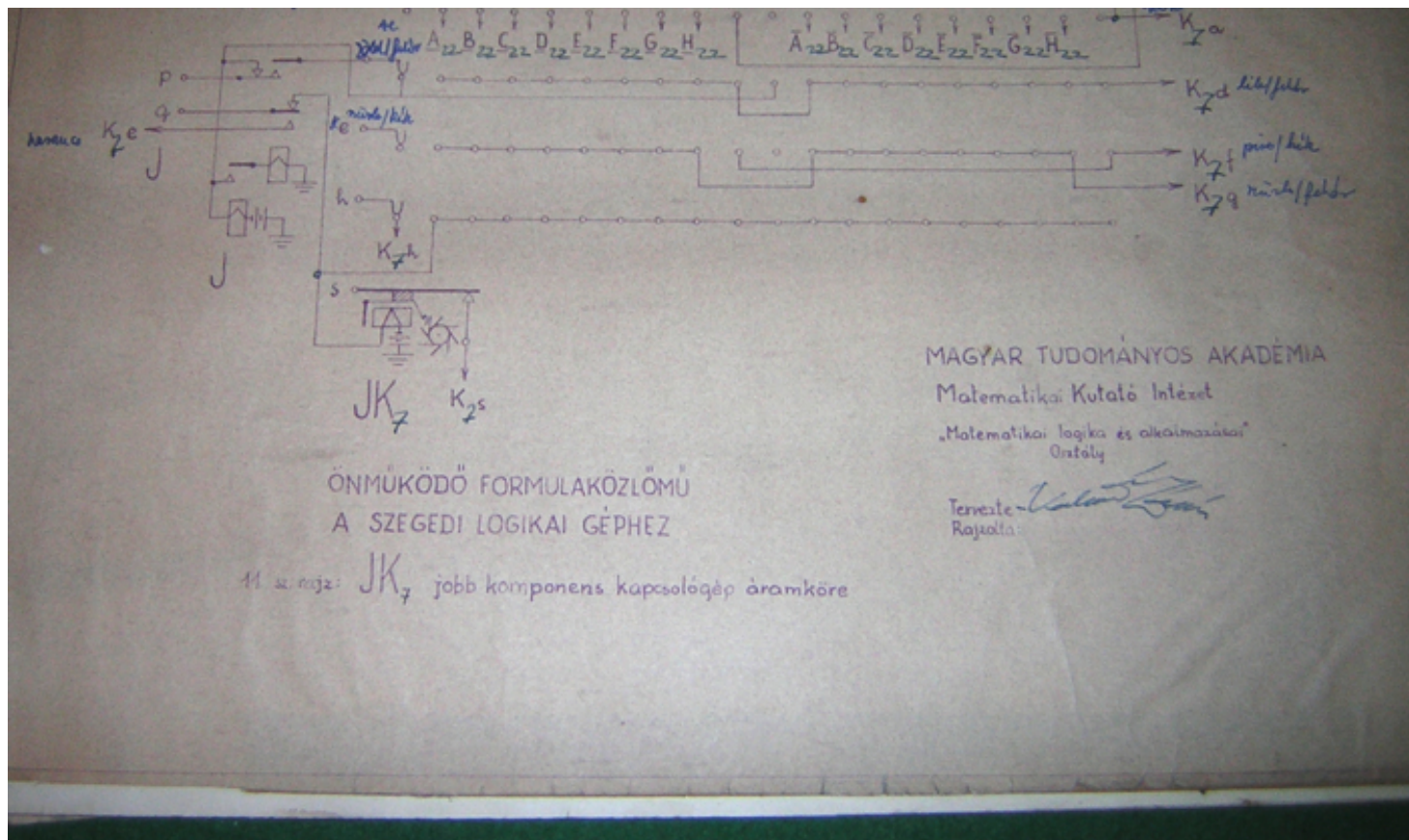
Tervrajzok formulavezérlésű géphez
