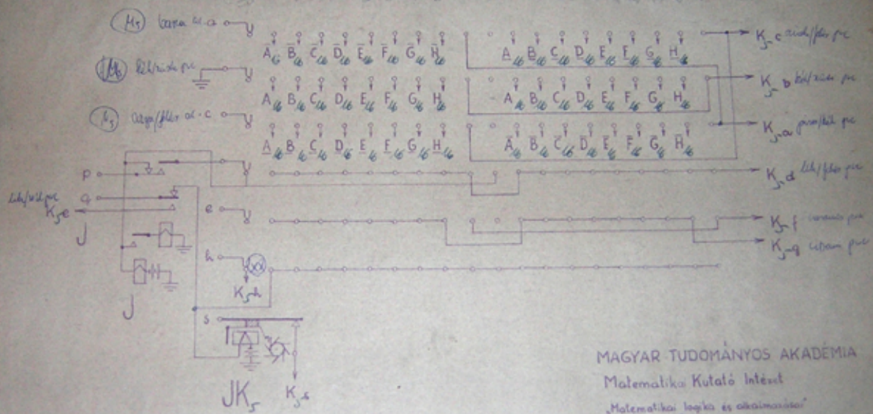
ÖNMŰKÖDŐ FORMULAKÖZLŐMŰ A SZEGEDI LOGIKAI GÉPHEZ 11. sz. rajz: JK_5 jobb komponens kapcsolólépcső áramkör
